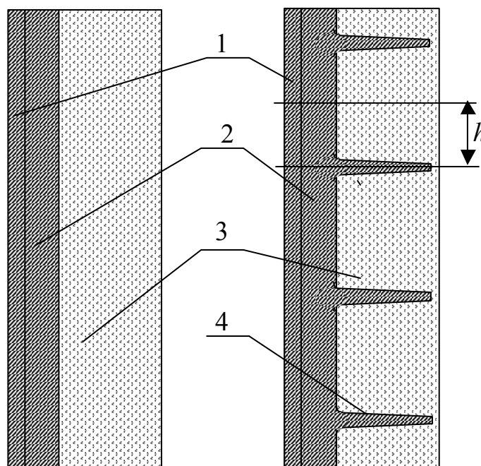
Рис. 1 Формы пластин.
