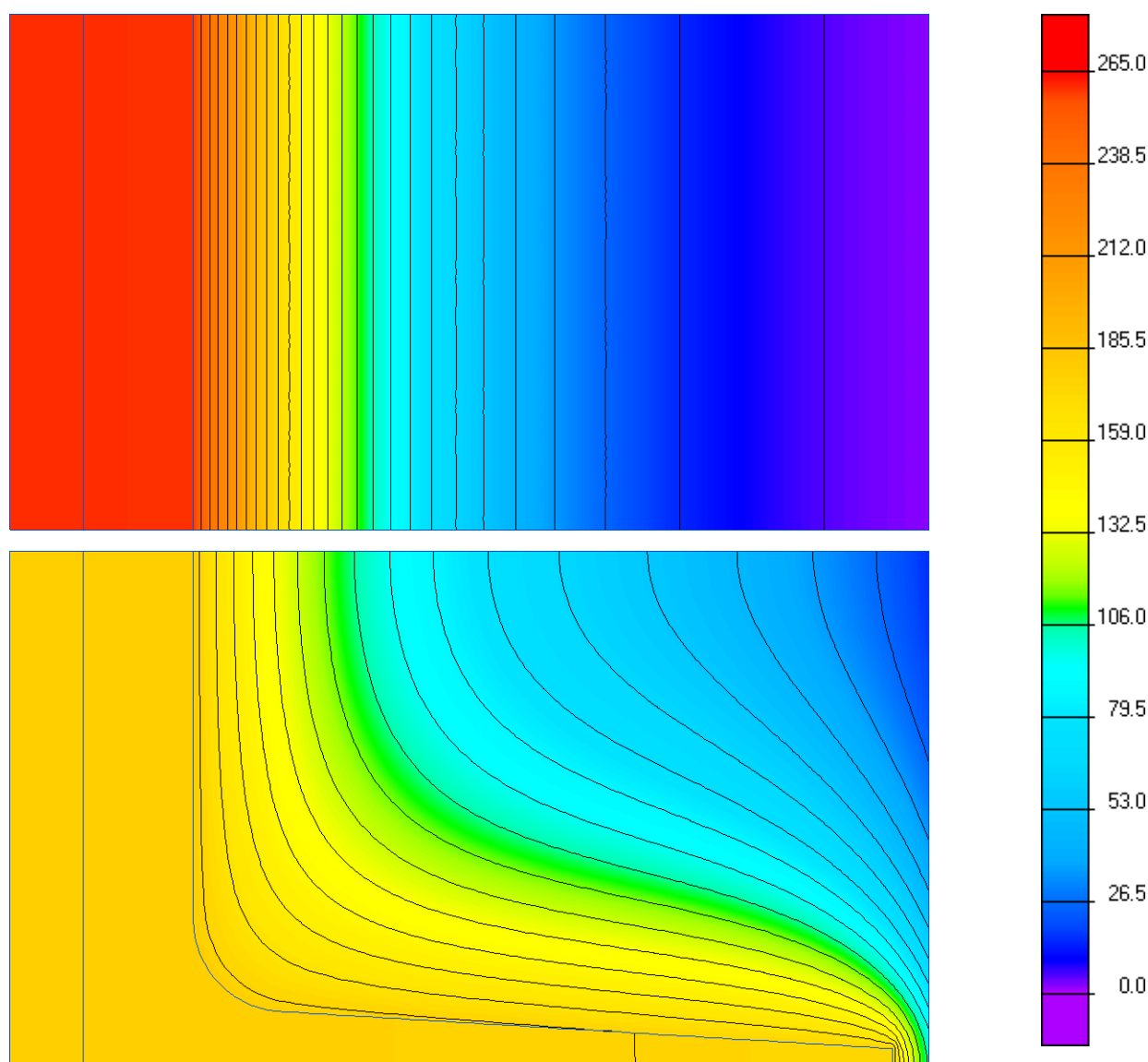
Рис. 2. Температурное поле плоской пластины (сверху) и оребренной пластины при h=56 мм
