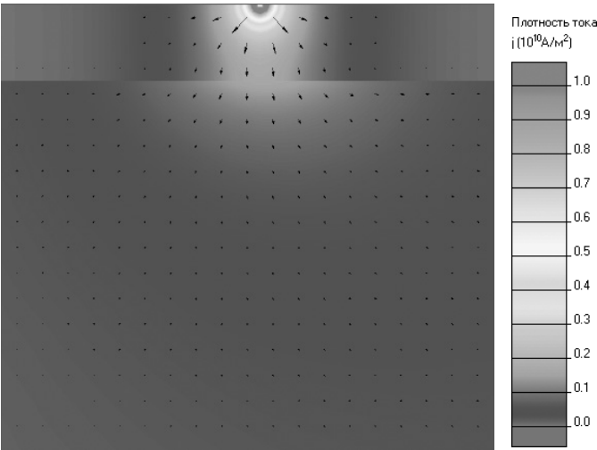
Рис. 11. Распределение плотности тока
