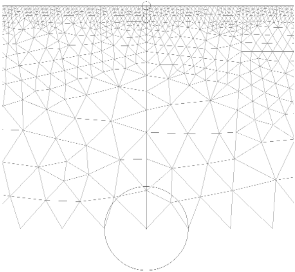
Рис. 10. Фрагмент сетки конечных элементов
