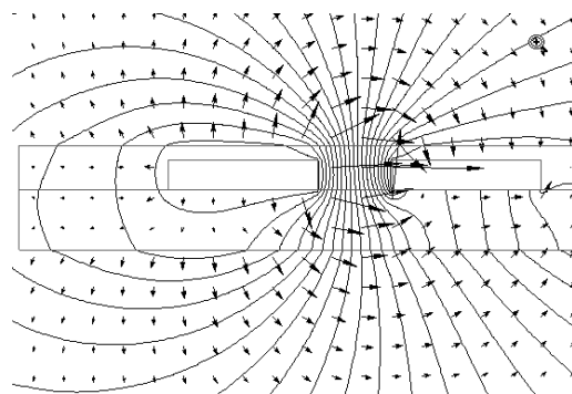
Рис. 7б. Векторы напряженности электрического поля
